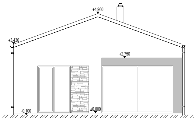
POHĽAD ZADNÝ
